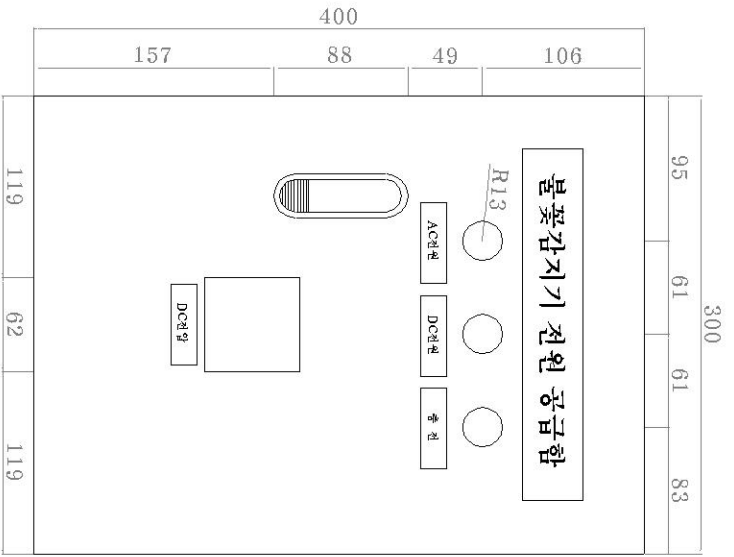
정면도
