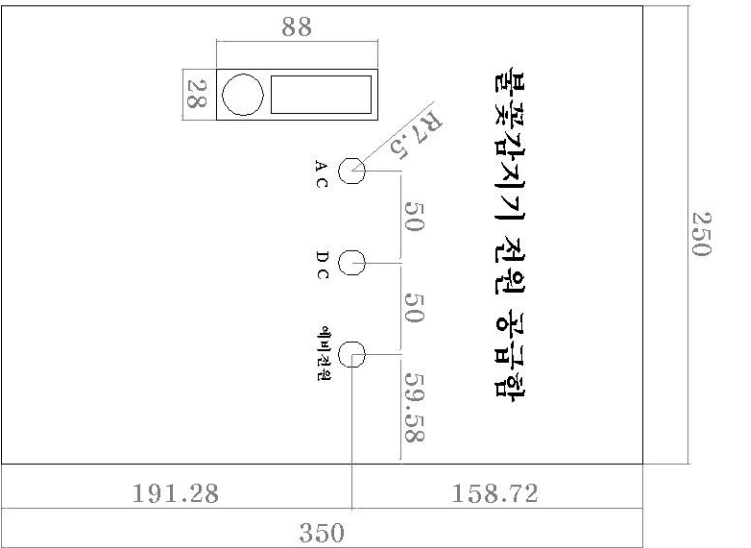
정면도
